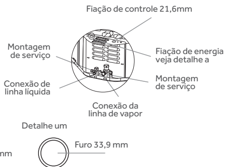
Fig.2 Dimensões
