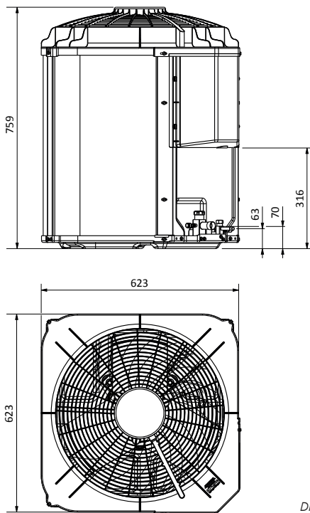
FIG. 7 - DIMENSIONAL UNIDADES CONDENSADORAS
