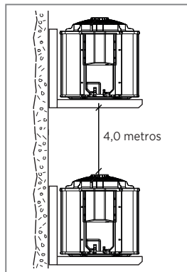
FIG. 6 - INSTALAÇÃO COM MÃO-FRANCESA
