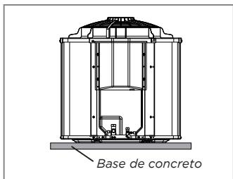
FIG. 4 - BASE RESISTENTE PARA INSTALAÇÃO
