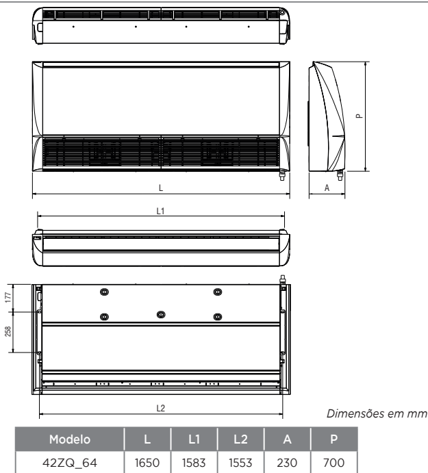
FIG. 8 - DIMENSIONAL UNIDADES EVAPORADORAS
