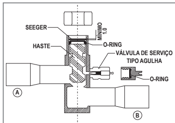
FIG. 21 - VÁLVULA DE SERVIÇO ABERTA
