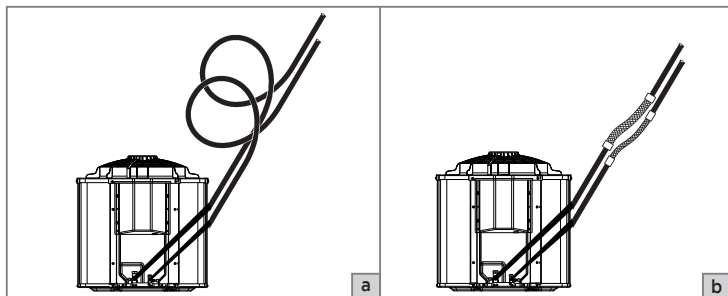
FIG. 18 - INSTALAÇÃO DOS LOOPS
