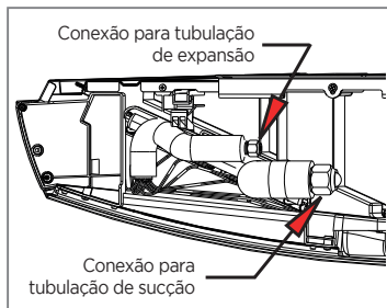
FIG. 19 - EX. CONEXÕES DE INTERLIGAÇÃO
