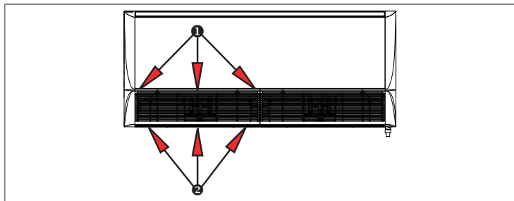
FIG. 13 - POSIÇÃO DOS PARAFUSOS PARA DESMONTAGEM DAS GRELHAS
