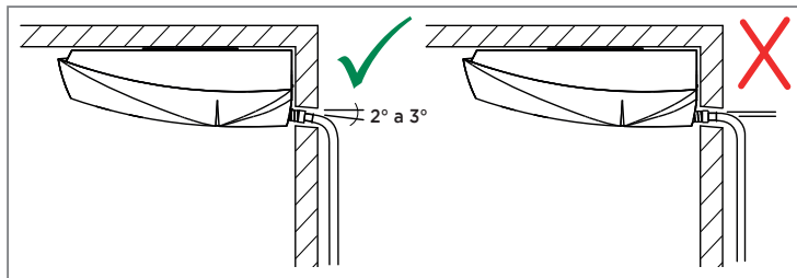
FIG. 15 - INCLINAÇÃO DRENAGEM
