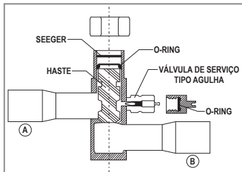
FIG. 20 - VÁLVULA DE SERVIÇO FECHADA
