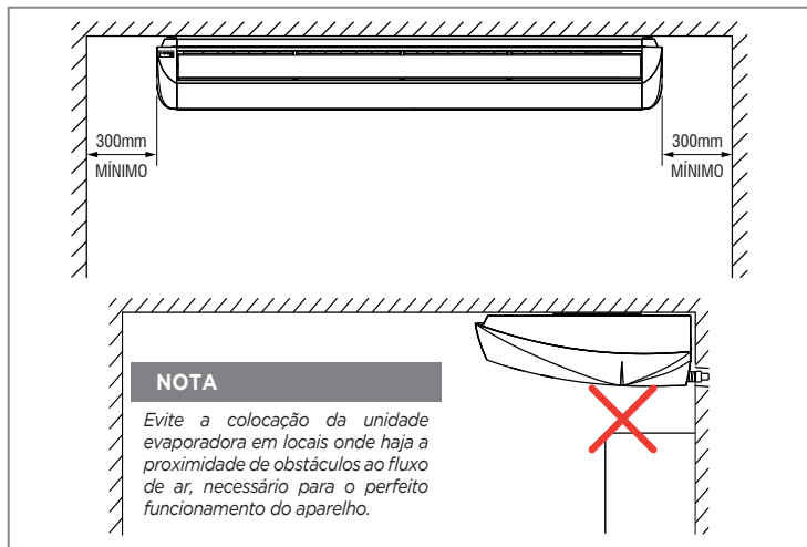
FIG. 9 - MONTAGEM DA UNIDADE
