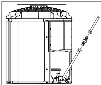
FIG. 25 - Instalação do kit sistema de expansão
