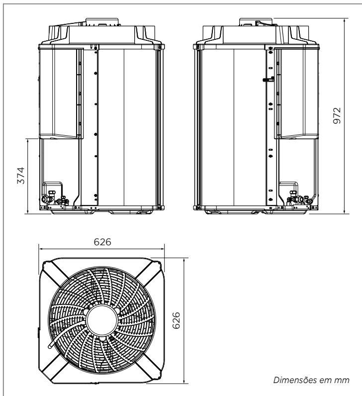
FIG. 6B - DIMENSIONAL UNID. CONDENSADORAS 38CQVF48 / 38CCVF54 / 38CQVF58
