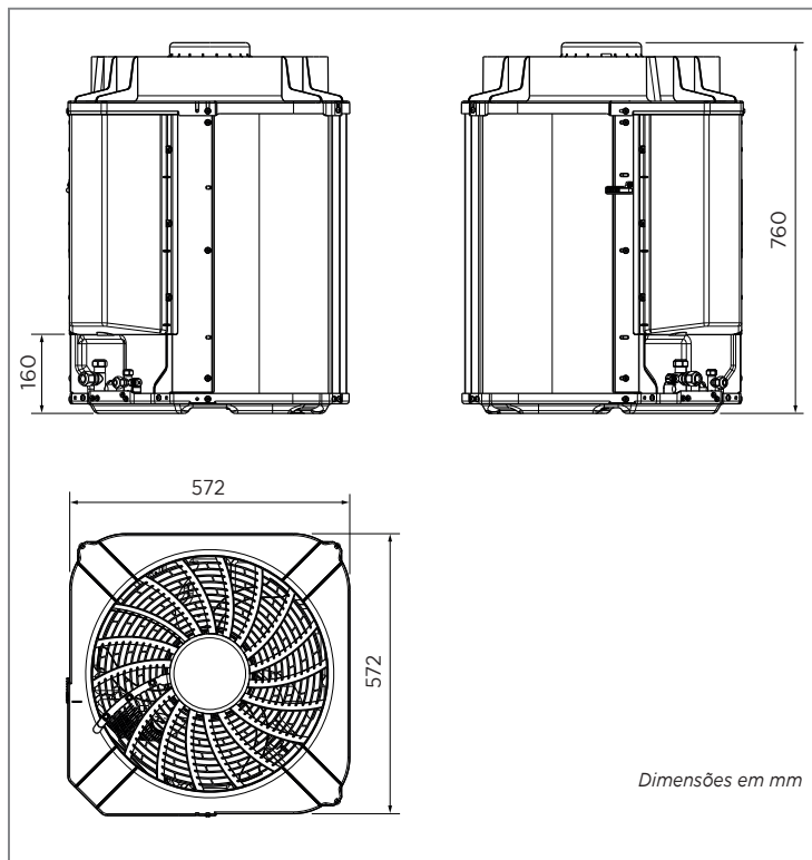
FIG. 6A - DIMENSIONAL UNID. CONDENSADORAS 38CCVF36 / 38CQVF36 / 38CCVF48
