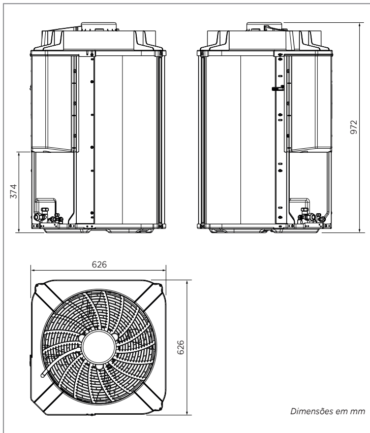
FIG. 9 - DIMENSIONAL UNIDADES CONDENSADORAS 38CQVF60
