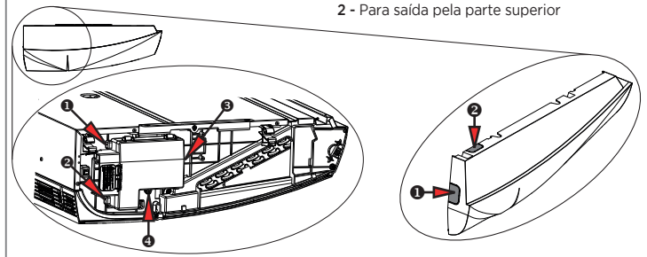
FIG. 25a - DETALHAMENTO CAIXA ELÉTRICA DA EVAPORADORA E CONEXÕES
