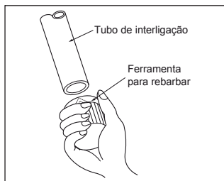
FIG. 54 - FERRAMENTA PARA REBARBAR
