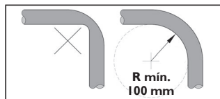
FIG. 62 - TUBULAÇÕES DE INTERLIGAÇÃO
