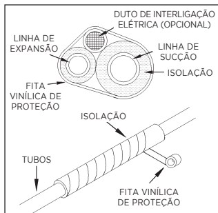
FIG. 63 - TUBULAÇÕES DE INTERLIGAÇÃO
