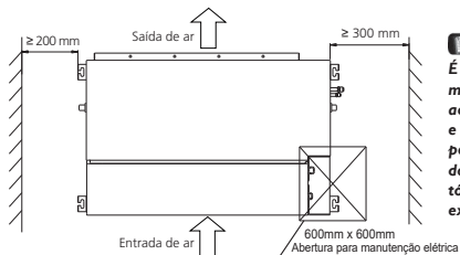
FIG. 36 - ESPAÇAMENTOS MÍNIMOS RECOMENDADOS PARA INSTALAÇÃO
