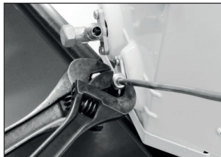
FIG. 58 - FIXAÇÃO DA PORCA
