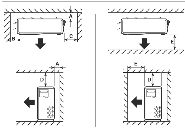
FIG. 8 - UNIDADES CONDENSADORAS
