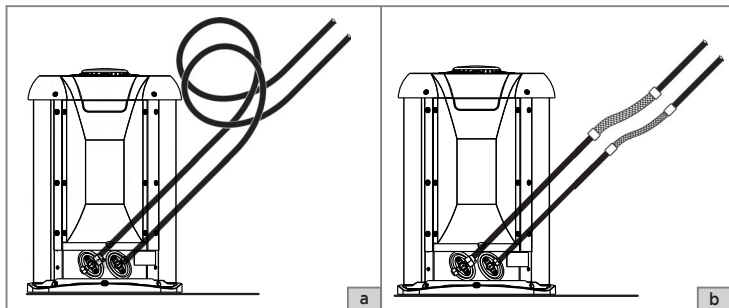
FIG. 21 - LOOP'S E TUBOS FLEXÍVEIS
