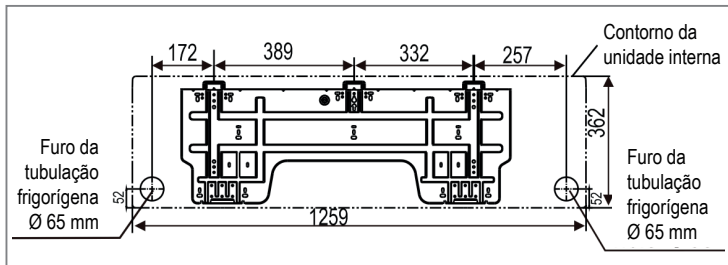
FIG. 19 - PLACAS DE MONTAGEM
