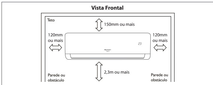
FIG. 14 - ESPAÇAMENTOS MÍNIMOS RECOMENDADOS
